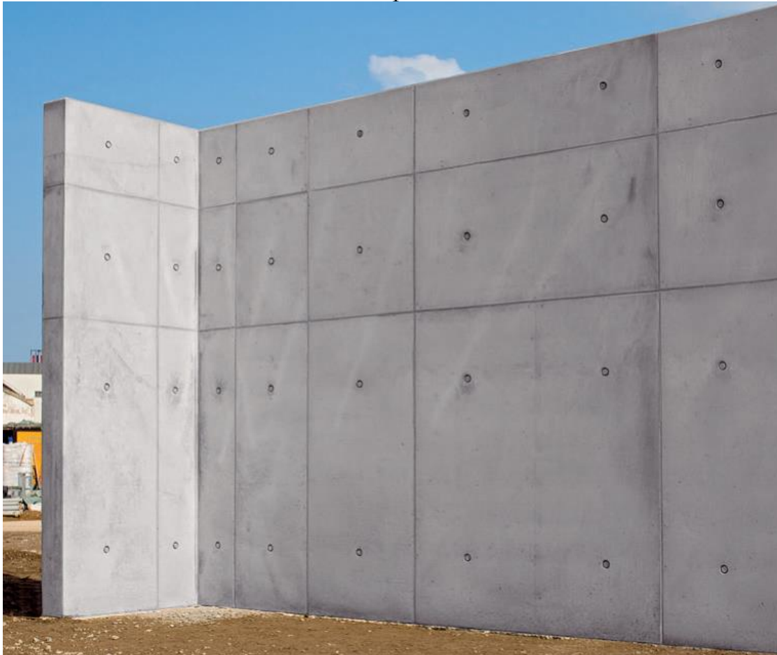
Esempio di realizzazione della finitura faccia-vista e chiusura dei fori dei tiranti previste in progetto
